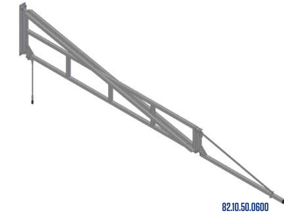
bras pivotant 4 mètres
